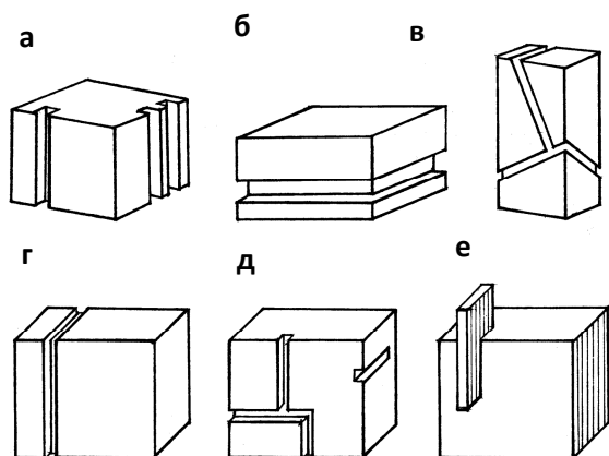
6–расм. Ҳажмийликнинг шакл сирти ва массасининг бўлиниш ҳолатларига боғлиқлиги: а–вертикал бўлиниш; б–горизонтал бўлиниш; г–яхлит бўлиниш; д–қисман бўлиниш; е–рельефли бўлиниш.
