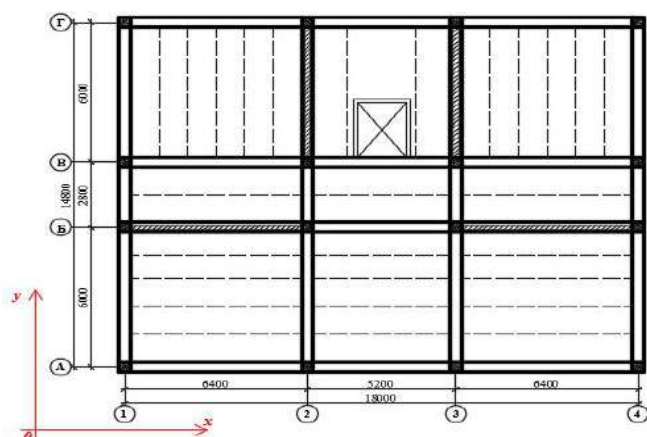
1-расм. Етти қават турар-жой биноси юк кўтарувчи конструкцияларининг фазовий кўриниши ва темир-бетон ёнма плиталарининг жойлашиши схемаси.
