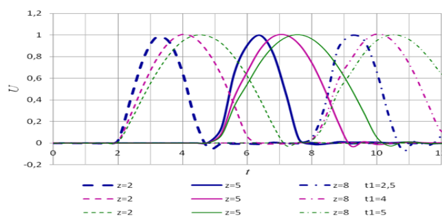
1-chizma. Ta'sir vaqtining turli qiymatlarida elastik sterjendagi ko'chishning vaqtdan bog'liq o'zgarishi ( \Omega = 0 )
