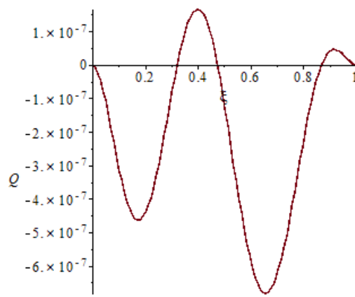
U_0^{(0)*}(x, t)
