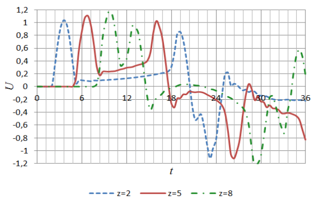
3-chizma. Aylanuvchi elastik sterjenda ko'chishning vaqt davomida o'zgarishi ( t_1=3 , \Omega=0,2 )
